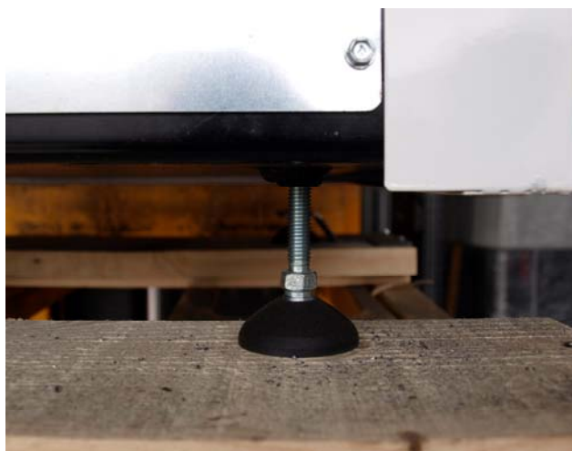
Slika 1: Nogice peći
